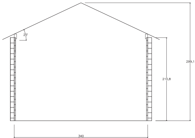
Schnitt / profile
