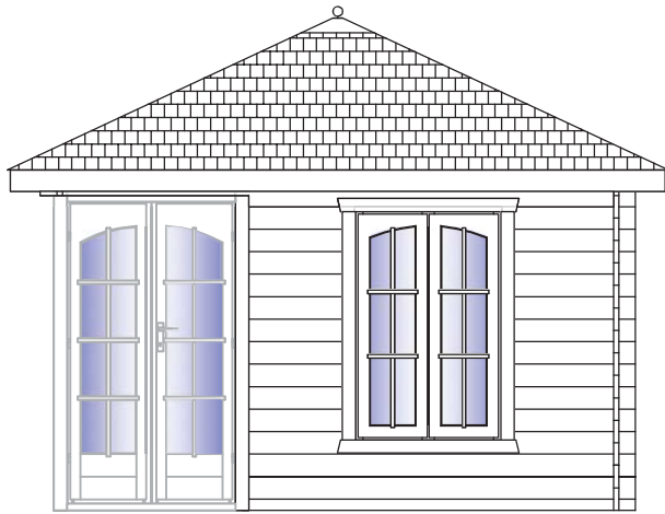
Ansicht vorne / front view
