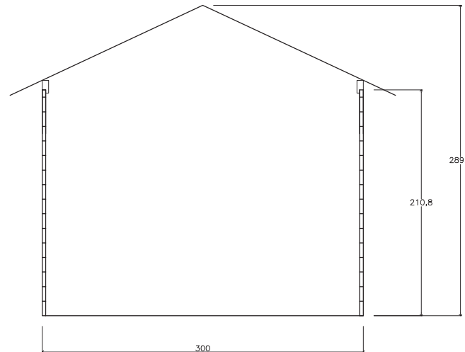
Schnitt / profile
