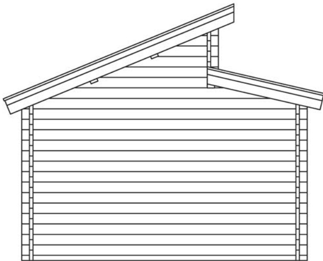
Ansicht hinten / back view
