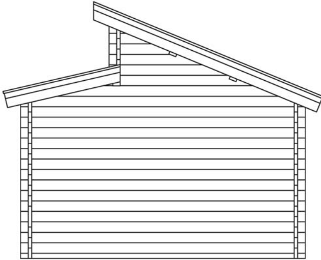
Ansicht vorne / front view
